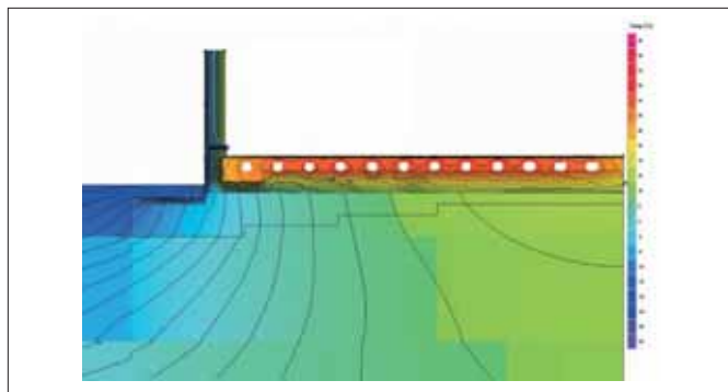
Połączenie konstrukcji płyty fundamentowej z podłogowym systemem grzewczym, uniemożliwia przenikanie wilgoci do betonu i stabilizuje temperaturę domu
